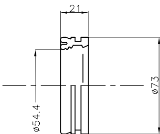
ゴムリング
